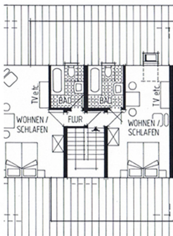
Doppelzimmer No. 5 & 6 im Dachgeschoss ca. 23-25 qm
