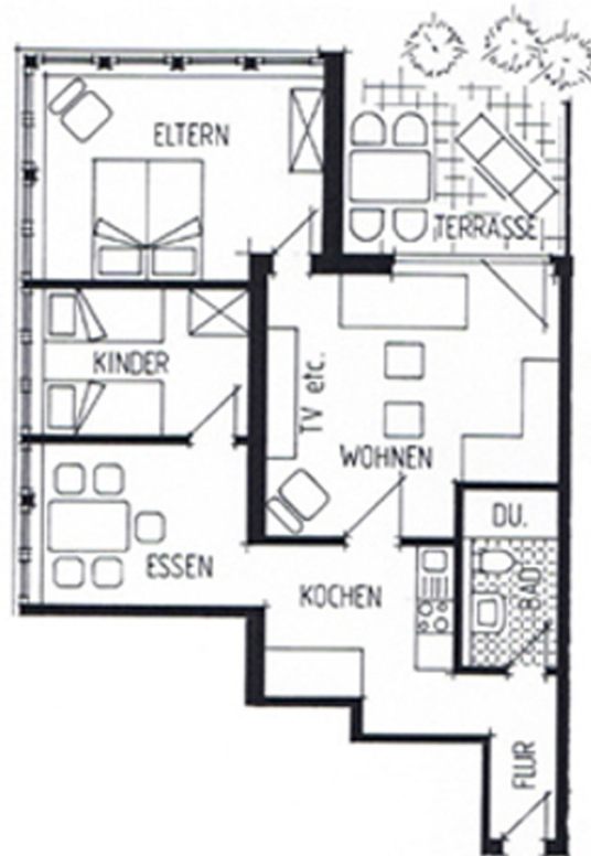
App. 1, 2 Schlafzimmer, 2 - 4 Personen, ca. 75 qm
